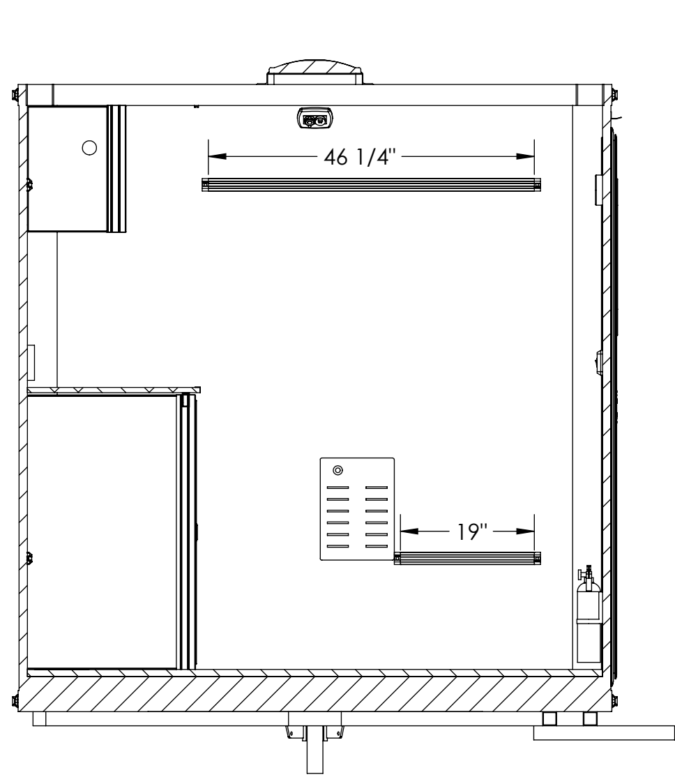
SECTION T-T SCALE 1 : 19
