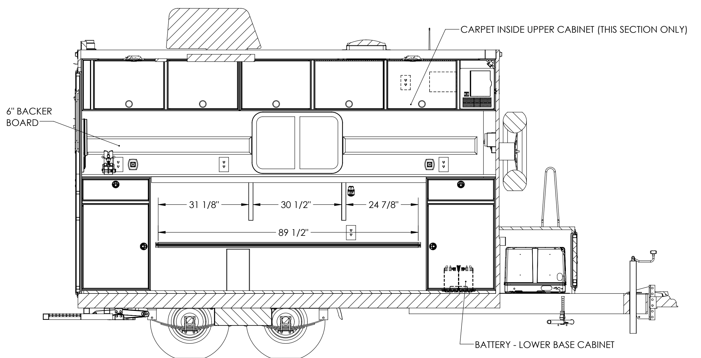
SECTION R-R SCALE 1 : 19
